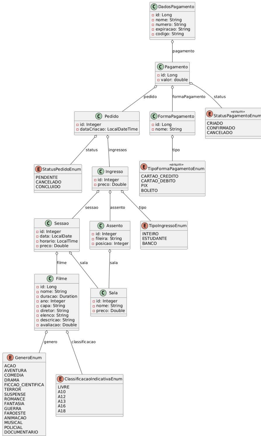
Diagrama de Classes - Ingresso
